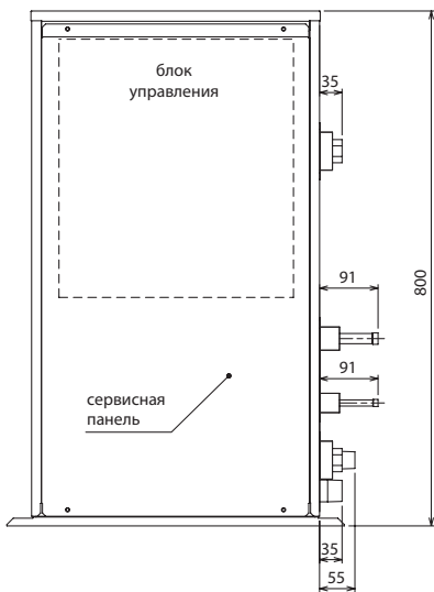
Вид спереди
