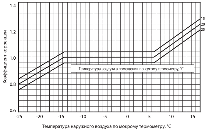
Коррекция теплопроизводительности
