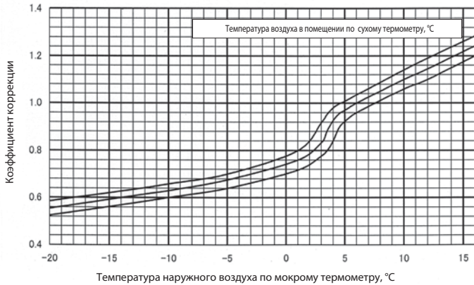
Коррекция теплопроизводительности
