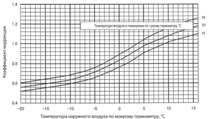
Коррекция потребляемой мощности в режиме нагрева
