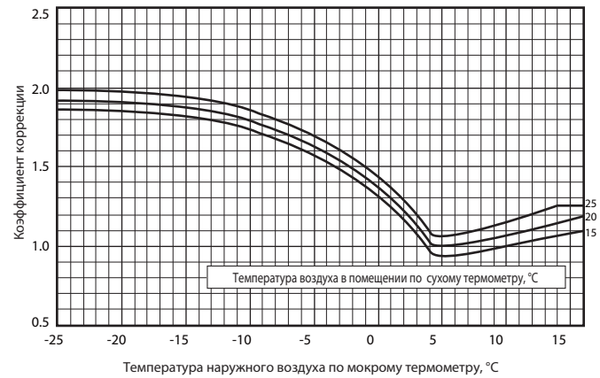
Коррекция потребляемой мощности в режиме нагрева
